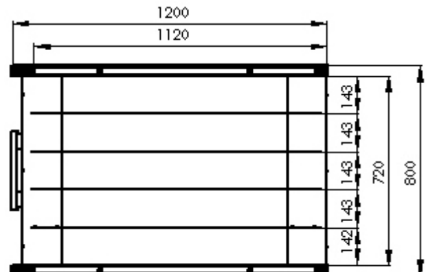
Schnitt Ebene 2
